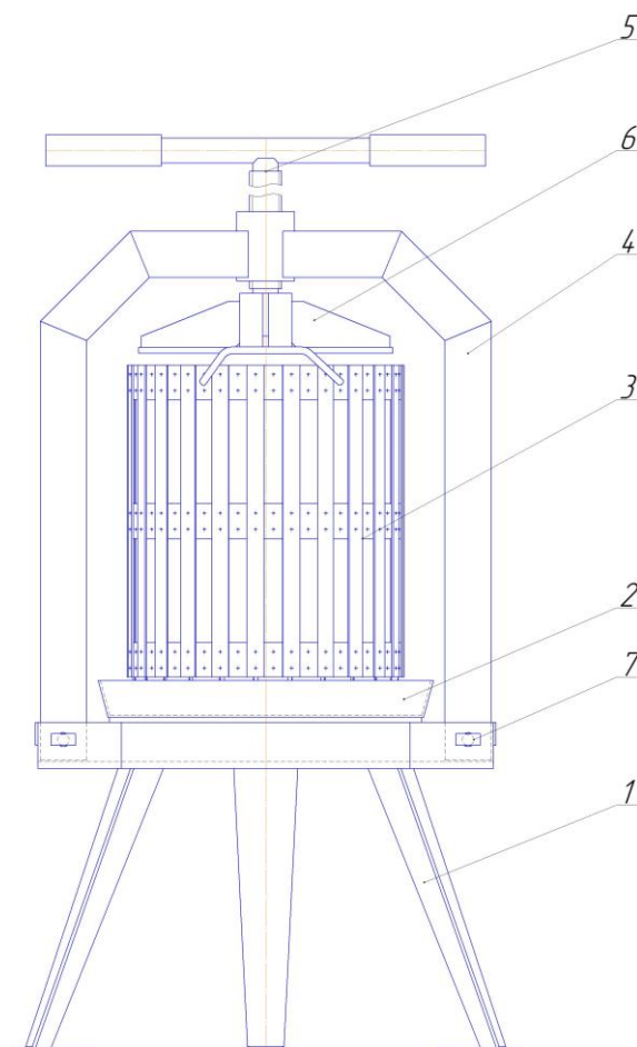
Рис. 1 Пресс
